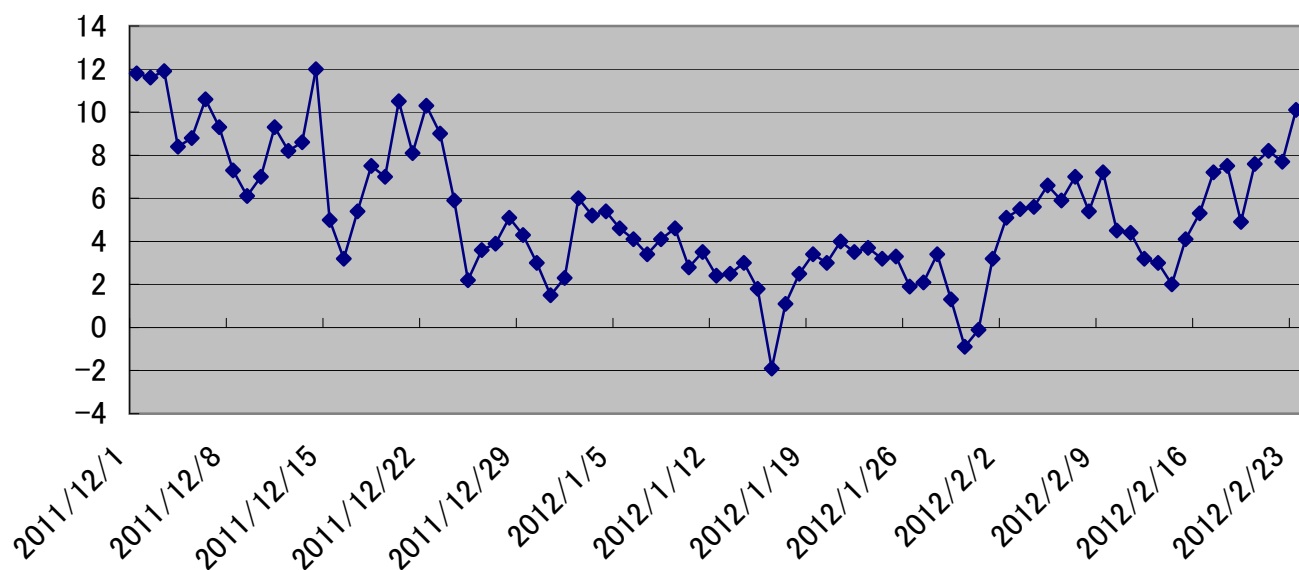
広島市平均気温推移
