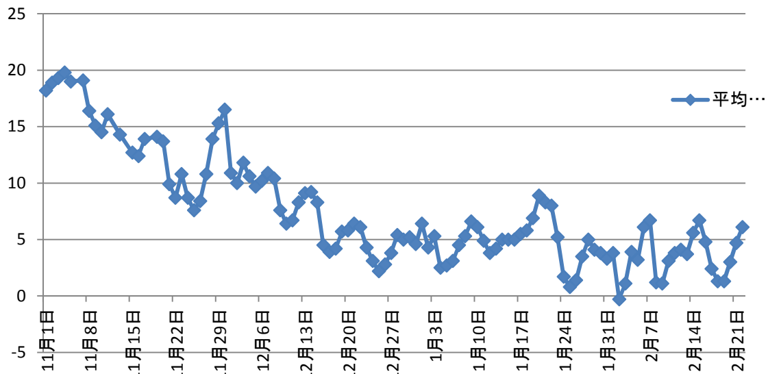
平均気温
